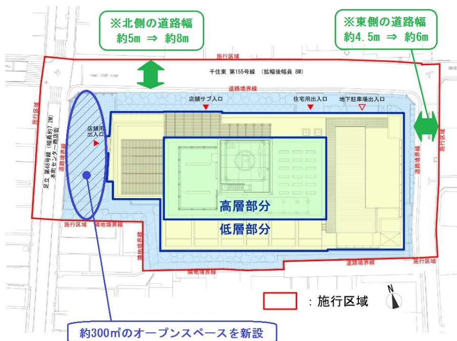
▲本事業計画の配置図
