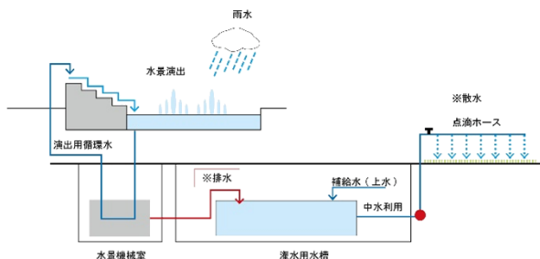
水量と灌水のハイブリット概念図
